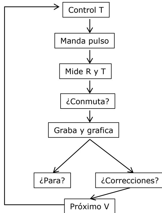
Figura 3-28: Diagrama del algoritmo utilizado para el experimento de la vida útil de los dispositivos.
