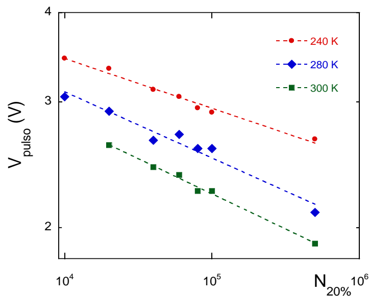
Figura 3-43: Curvas V-N a diferentes temperaturas para un \alpha de 20%. Las líneas punteadas corresponden a la regresión lineal realizada según la ecuación (10). Al igual que en los ensayos de fatiga mecánica, disminuir la temperatura mueve las curvas hacia valores de voltaje mayores.
