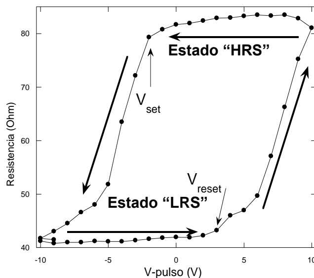
Figura 2-5: RSHL característico para la resistencia de un contacto de una muestra de YBCO con electrodos de Pt. Se pueden distinguir claramente los estados de resistencia alta (HRS), baja (LRS) así como los voltajes críticos de V_{set} y V_{reset} y las zonas de transición entre los ellos.
