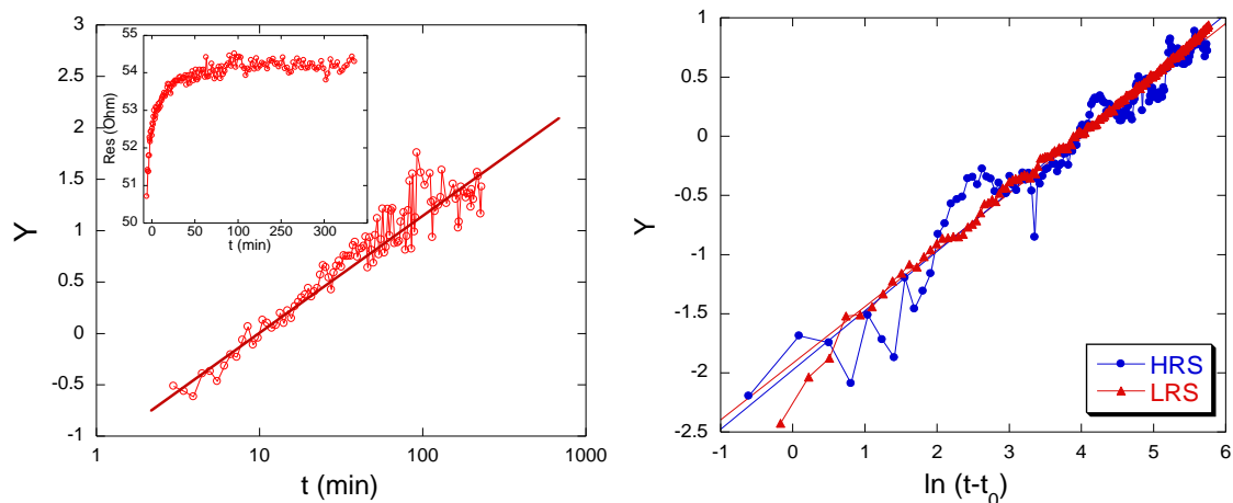
Figura 3-20: Izquierda: Linealización según la ecuación 6 de la evolución temporal de la variación resistiva de una junta de Pt/YBCO a una temperatura fija (123 K) luego de haber producido la CR. En el inset se muestra la evolución de la resistencia en función del tiempo para el mismo set de datos. Derecha: se muestra como la ecuación 6 describe adecuadamente el comportamiento de la relajación de ambos estados de resistencia obtenidos.
