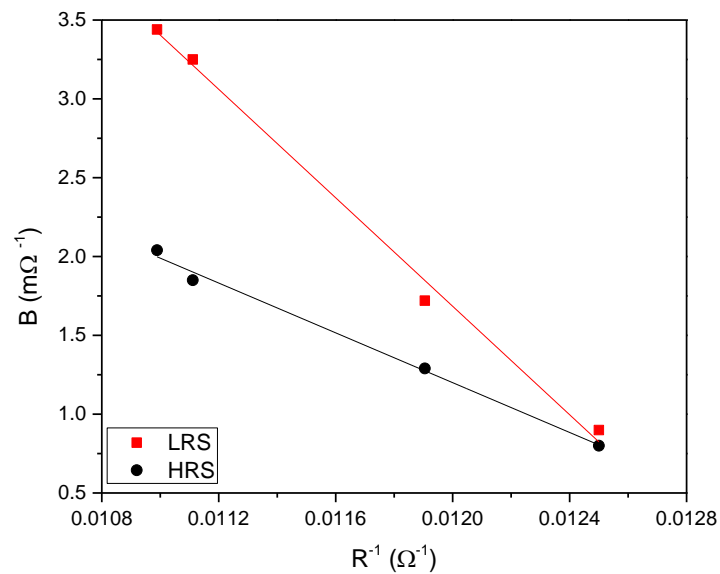
Figura 3-54: Relación existente entre el coeficiente B de la ecuación 11 y la inversa de la resistencia medida a 4 terminales para las temperaturas estudiadas.
