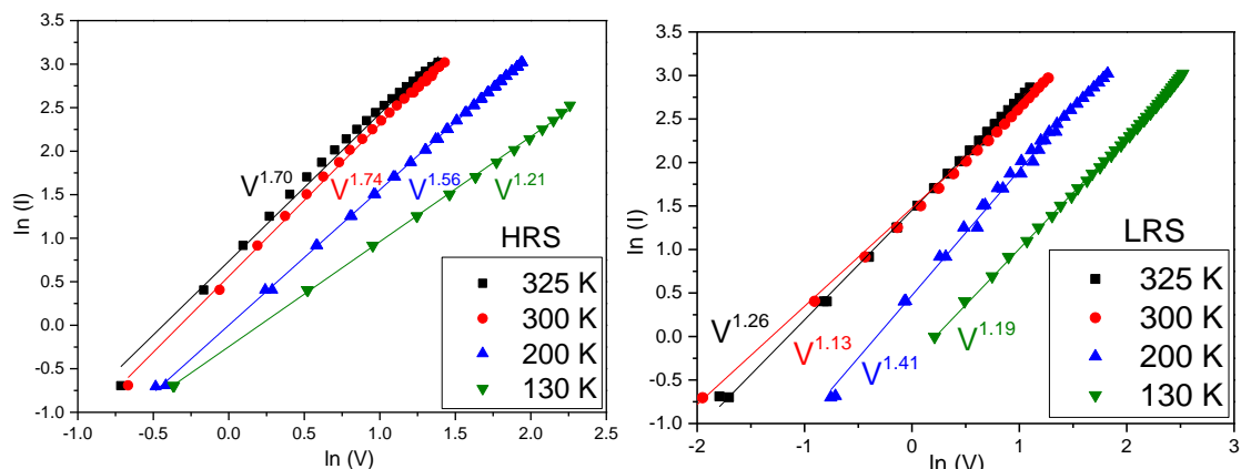
Figura 3-51: Izquierda (derecha) curvas \ln(I) vs. \ln(V) para el estado HRS (LRS) de la juntura Ag/LSCO a diferentes temperaturas.
