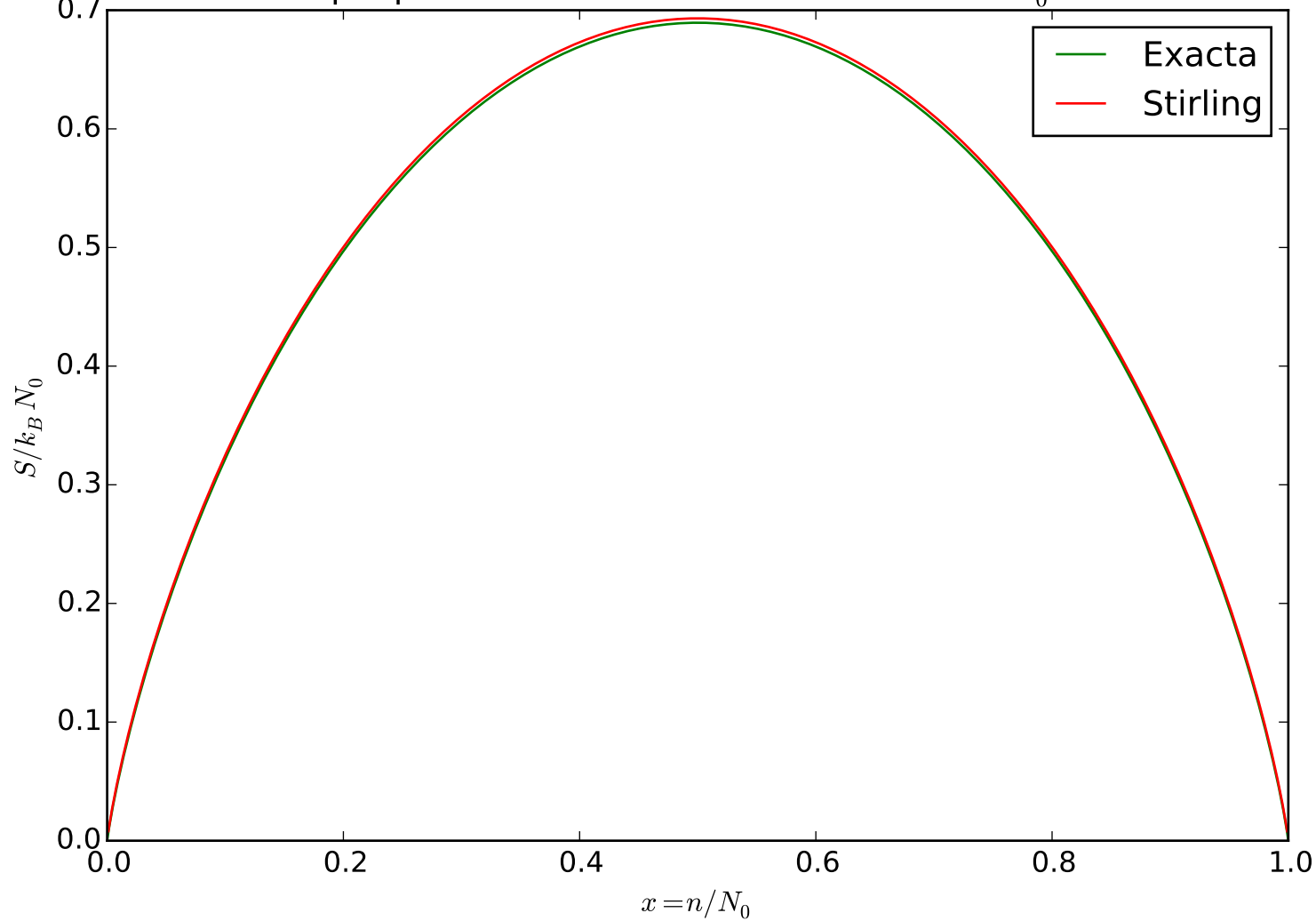
Entropía para un sistema de dos niveles con N_0 = 1000
