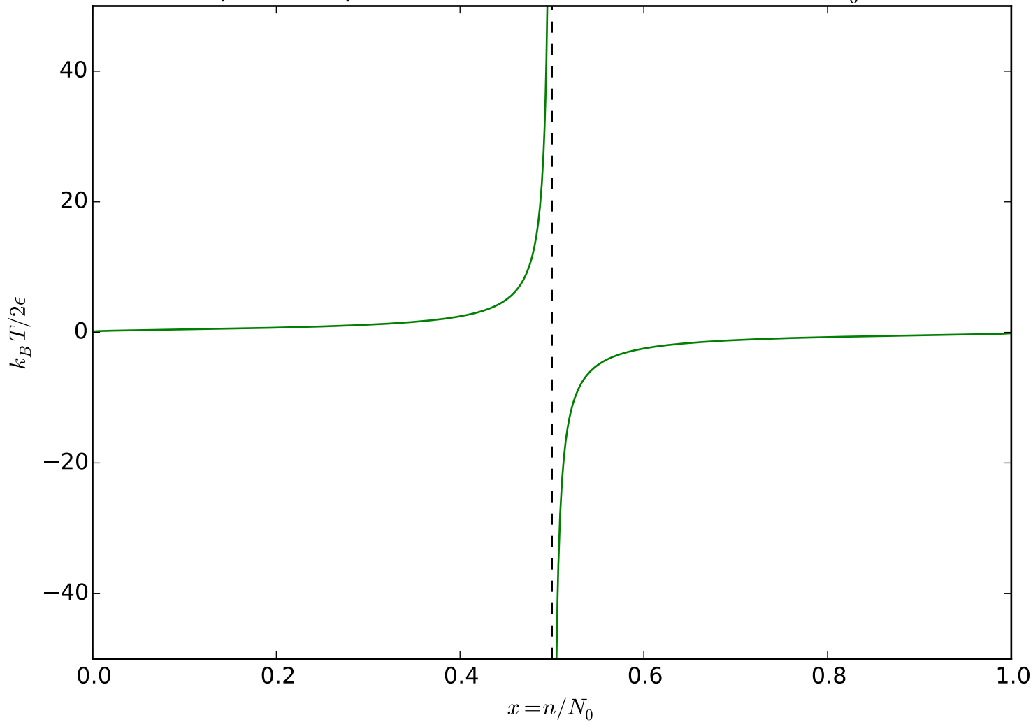
Temperatura para un sistema de dos niveles con N_0 = 1000
