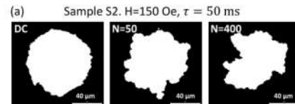
Evolución de un dominio magnético bajo la aplicación de N pulsos alternos de amplitud grande y baja frecuencia.
