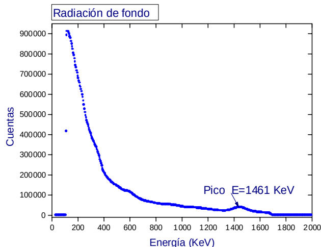
Figura3: Espectro de la radiación de fondo
