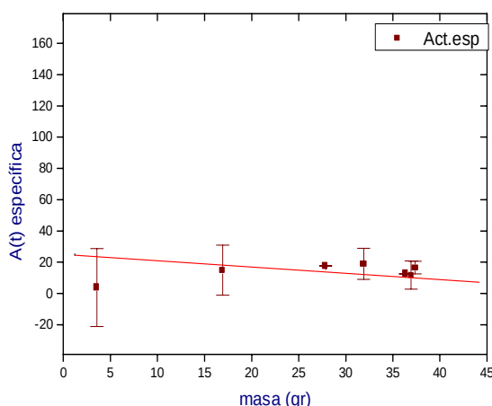
Figura5: Actividad específica en función de la masa. La curva roja corresponde al ajuste lineal de los datos.
