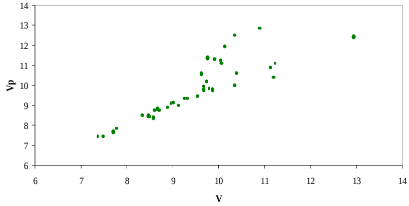
Figura 3: Comparación de las magnitudes verdes obtenidas con nuestros filtros (V), y las magnitudes standar (Vp).
