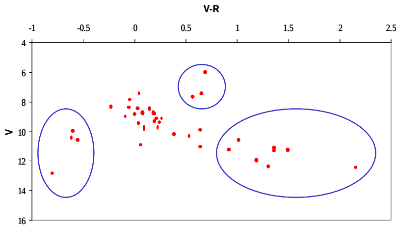
Figura 5: Diagrama de magnitud aparente vs. color para el cúmulo NGC 3532. Las regiones marcadas son serán tenidas en cuenta para el ajuste de secuencias.
