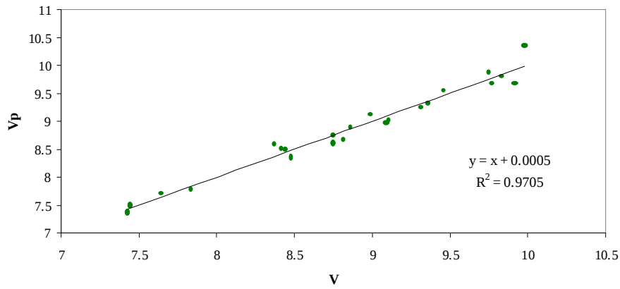
Figura 4: Comparación de las magnitudes verdes obtenidas con nuestros filtros (V), y las magnitudes standar (Vp), sin tener en cuenta las de magnitud mayor a 10.
