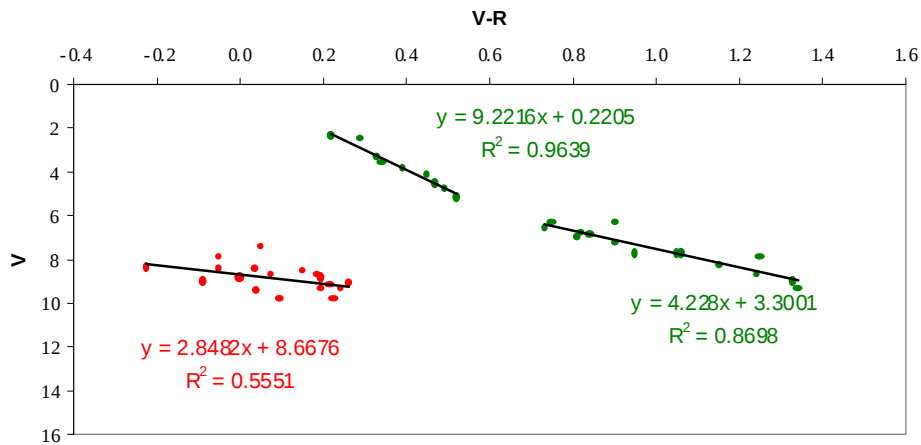
Figura 5: Diagrama de magnitud aparente vs. color para el cúmulo NGC 3532. Las regiones marcadas son serán tenidas en cuenta para el ajuste de secuencias.
