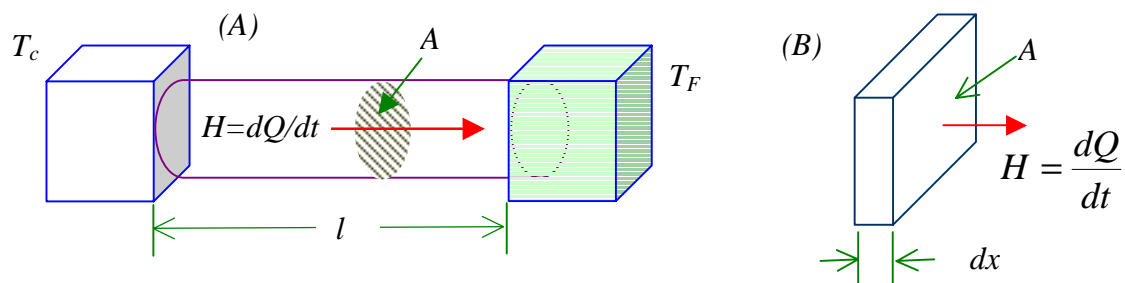
Figura 1. (A) Transmisión del calor a lo largo de una barra de materia, asilada por los lados laterales, de longitud l con un extremo caliente ( T_C ) y el otro frío ( T_F ). (B) Transmisión de calor a través de un elemento de materia de espesor infinitesimal dx .
