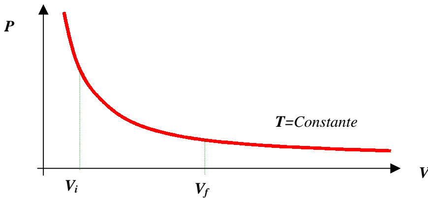
Fig. A2- Expansión reversible, isotérmica, de un gas ideal.
