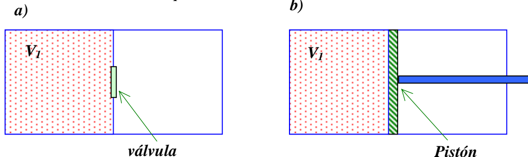
Fig. A1- Expansión libre de un gas ideal. a) Proceso irreversible, el gas originalmente esta en la mitad izquierda, mientras que la derecha está vacía. Al abrir la válvula, el gas ocupa ambos recipientes. b) Proceso equivalente al de la izquierda, pero a través de un proceso reversible.
