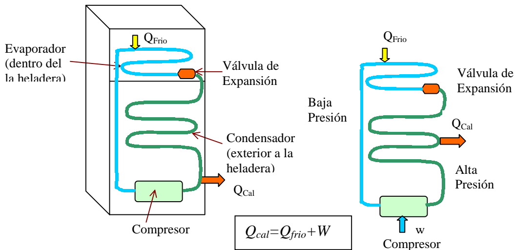
Figura 8: Componentes básicas de un refrigerador domestico.
