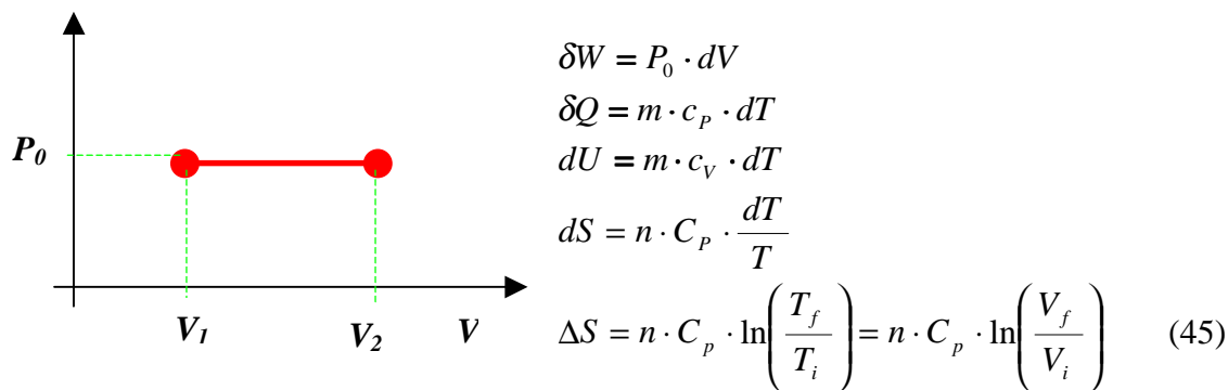
Figura 5: Proceso Isobárico.
