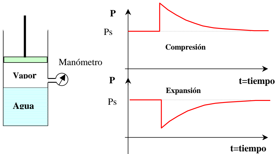
Figura 1. Comportamiento de un vapor.
