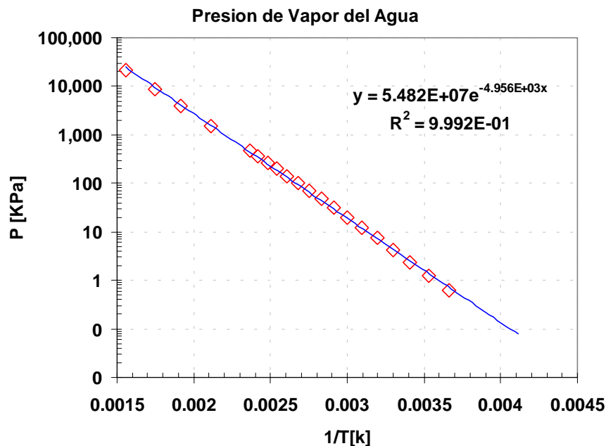
Figura 8: Presión de vapor del agua en K Pa como función de 1/T [K], para temperaturas comprendidas entre 0^\circ\text{C} y 370^\circ\text{C} . La dependencia mostrada claramente indica que la dependencia de la Presión de vapor sigue la tendencia predicha por la ecuación de Clausius-Clapeyron, ec.(47").
