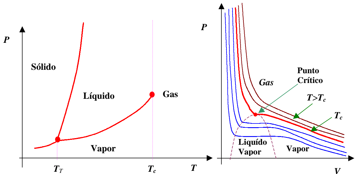
Figura 2. Diagrama esquemático de los distintos estado de una sustancia pura. A la izquierda, representamos P en función de T . Los ejes coordenados representan la presión y temperatura. Las líneas continuas representan estados de equilibrio en la que pueden existir dos o más fases de dicha sustancia. A la derecha, representamos P en función de V . Los punto de las isothermas de T < T_c , describen las propiedades del vapor. Dentro de la campana, coexisten las dos fase, liquido y vapor. El punto de la isoterma crítica en el que coexisten el líquido y el vapor se llama punto crítico. El valor de la presión y volumen (para 1 mol) definen los valores de Presión Crítica ( P_c ) y Volumen Crítico ( V_c ).
