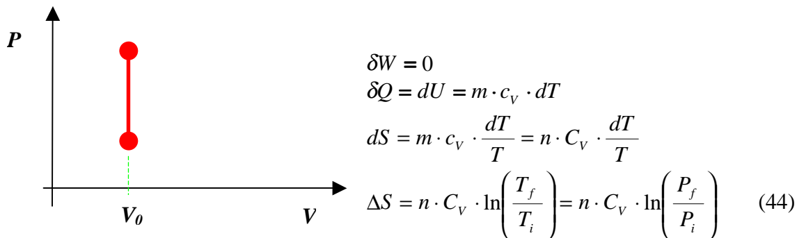
Figura 4: Proceso Isocórico.
