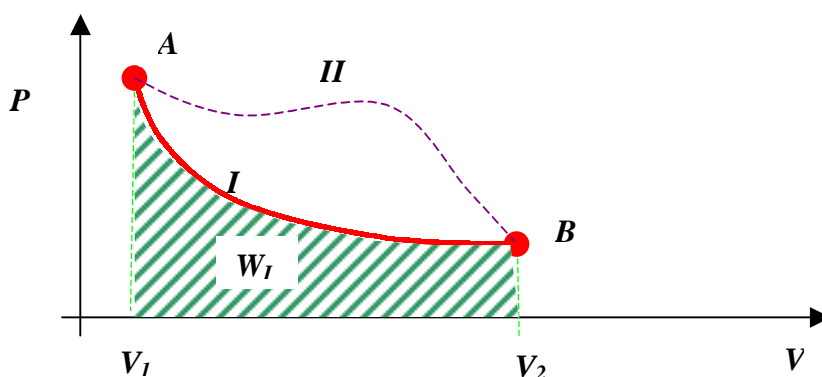
Figura 3: Trabajo realizado por el sistema para ir del estado A a otra B por dos trayectoria distintas I y II. Se ve que el trabajo para ir de A a B depende de la trayectoria. Por lo tanto el trabajo, al igual que el calor, no son variables de estado.
